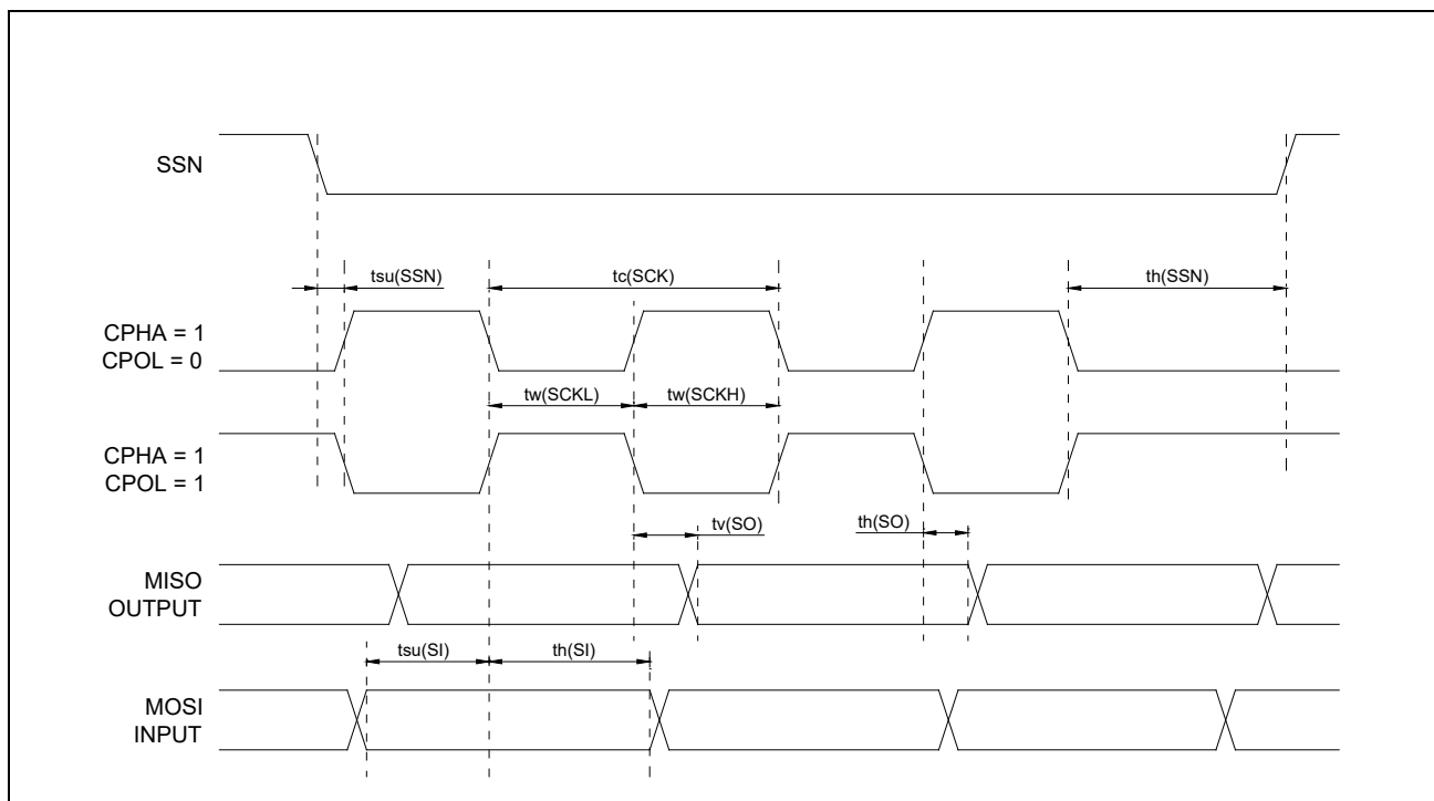
图 7-6 SPI 时序图 (从机模式 cpha=1)
