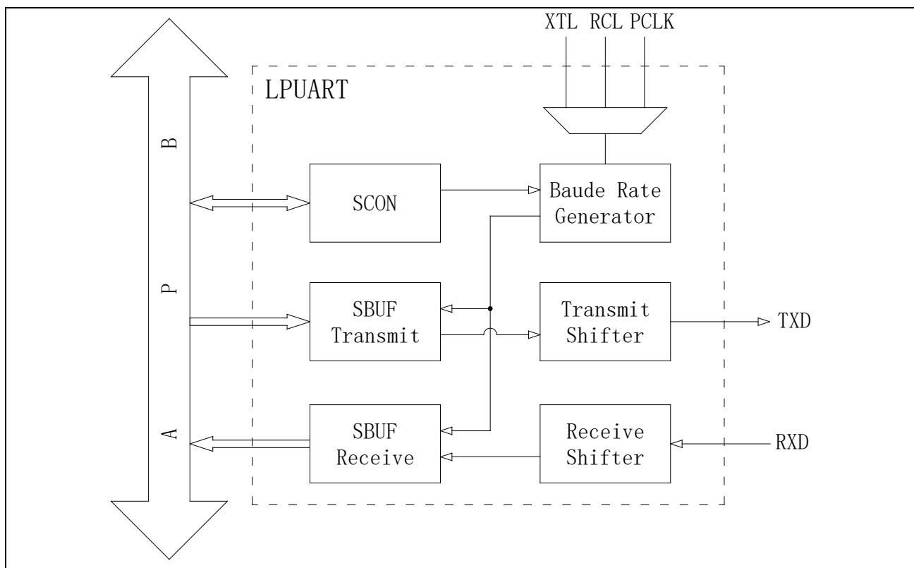
图 22-1 结构框图
