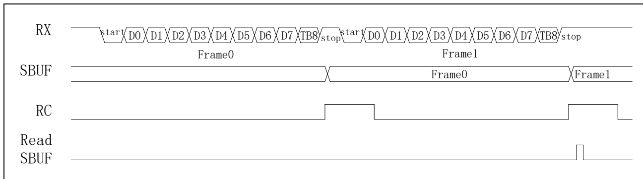
图 21-13 接收缓存
