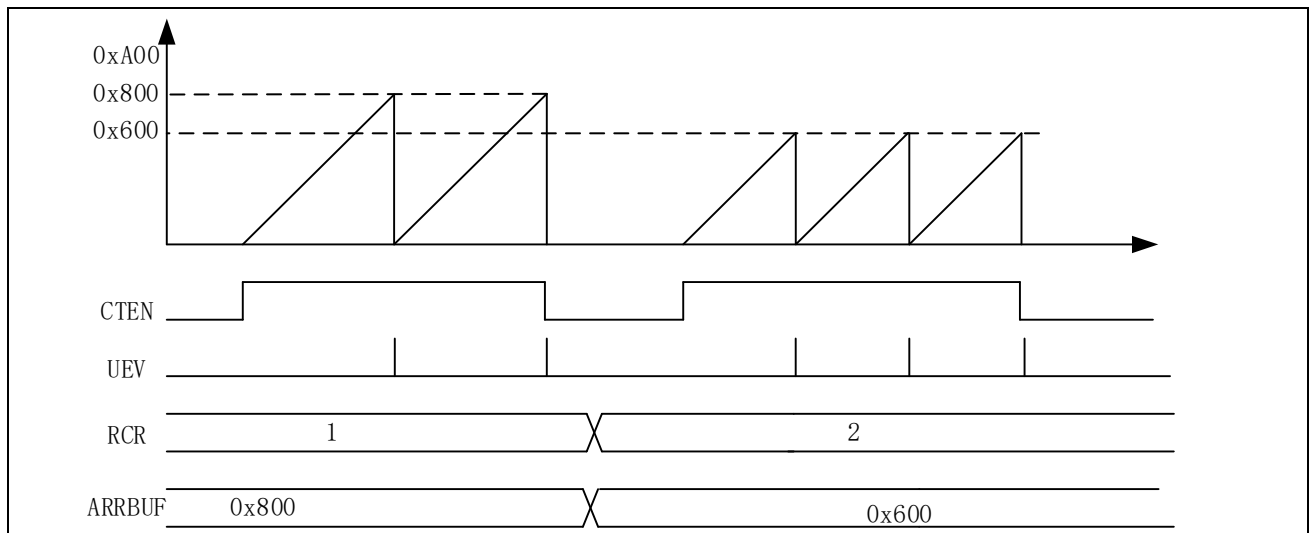
图 14-44 锯齿波上计数单脉冲模式
