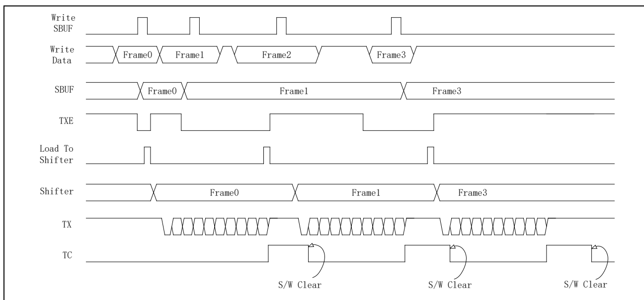
图 21-14 发送缓存
