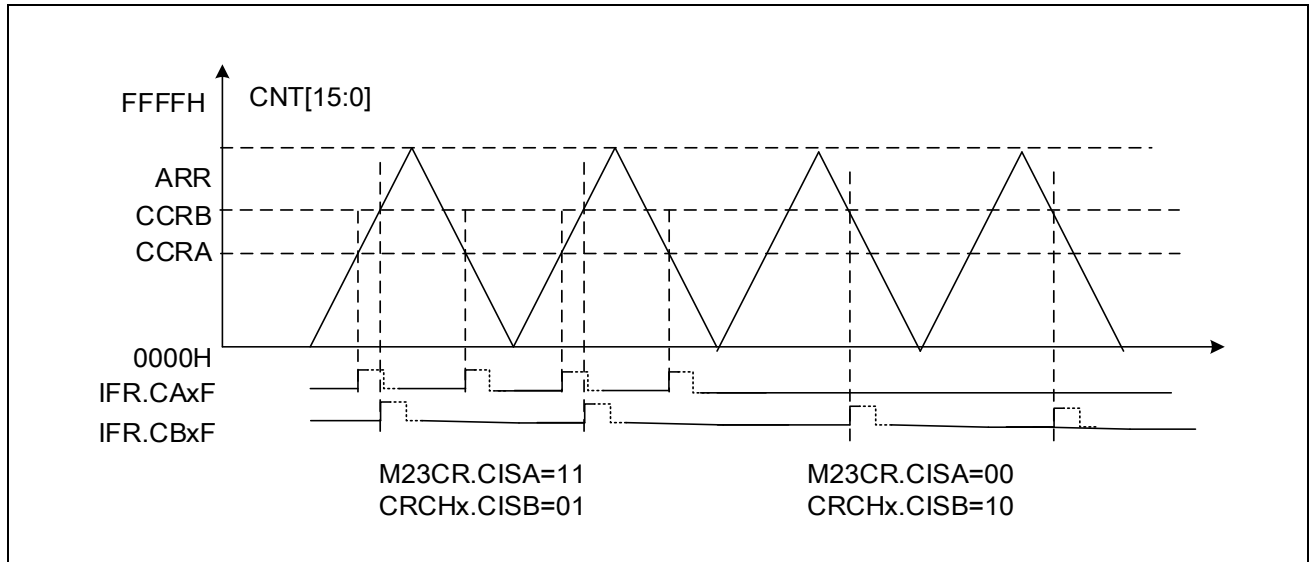
图 14-46 中断示意图
