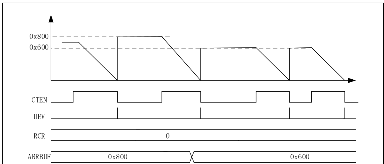
图 14-45 锯齿波下计数单脉冲模式
