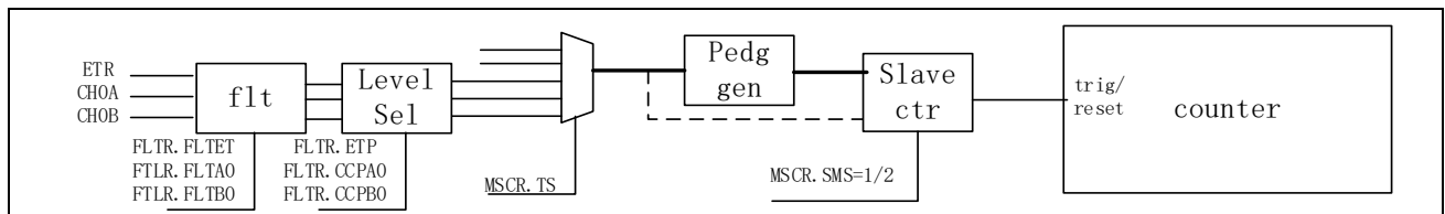
图 14-53 触发和复位功能
