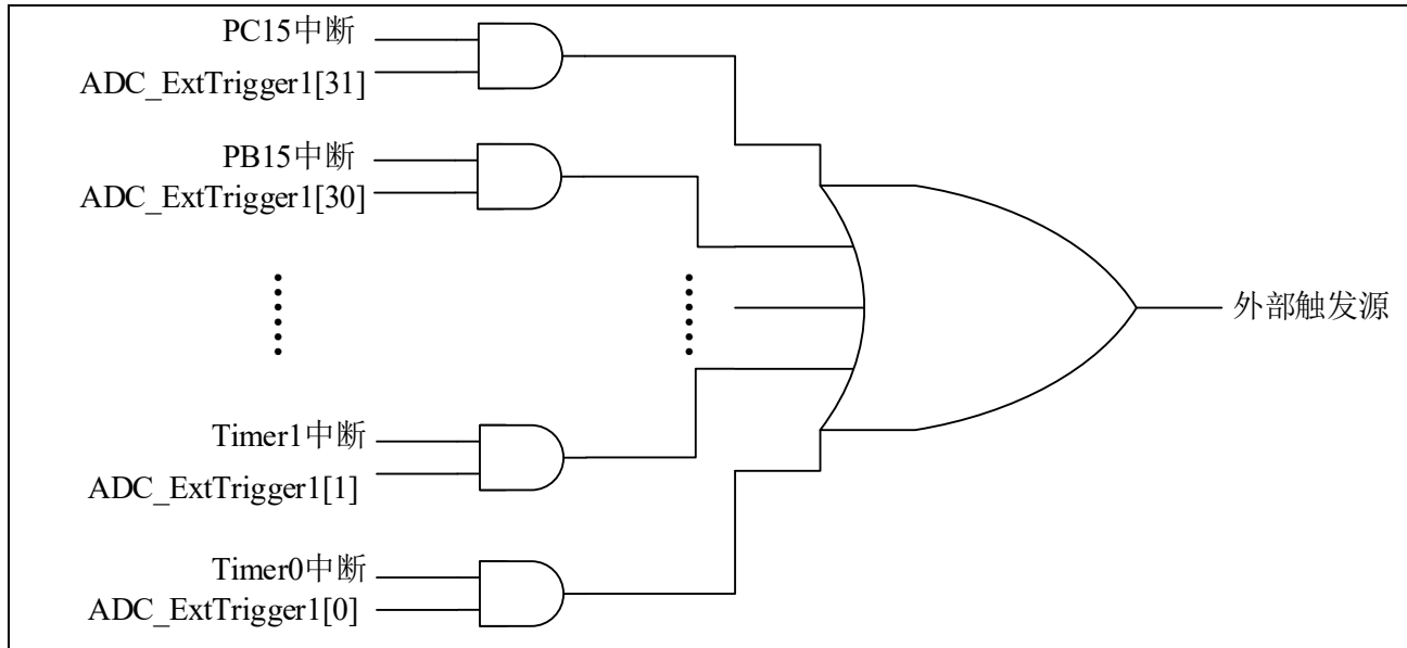
图 27-8 ADC 插队扫描转换外部触发源示意图
