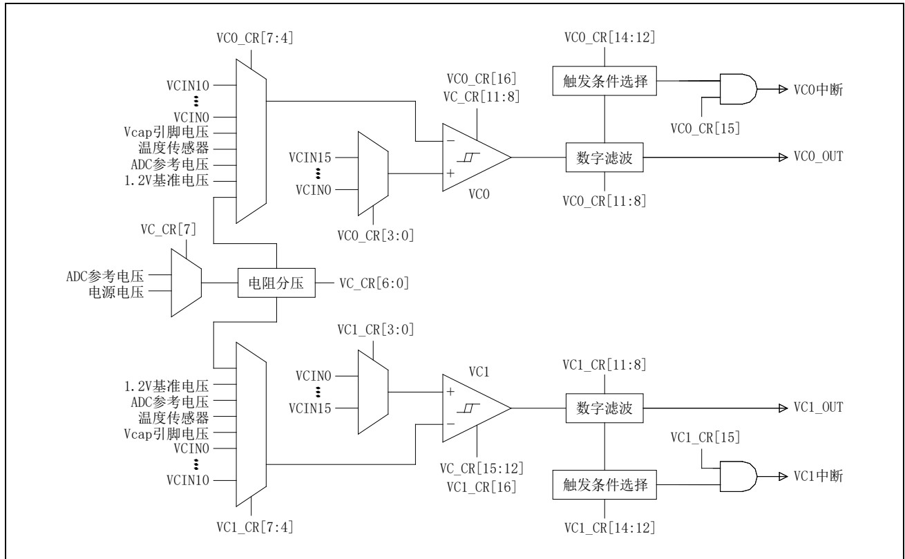
图 28-1 VC 框架图
