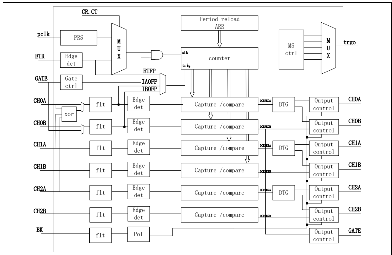
图 14-2 TIM3 框图
