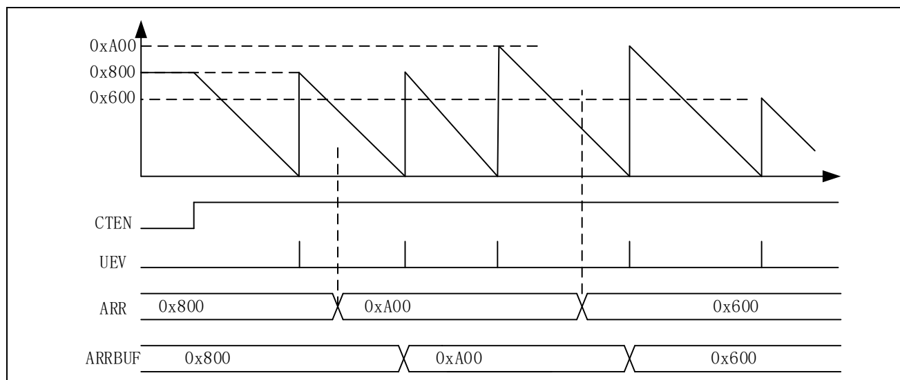
图 14-28 锯齿波模式下计数缓存使能
