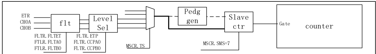
图 14-52 门控功能
