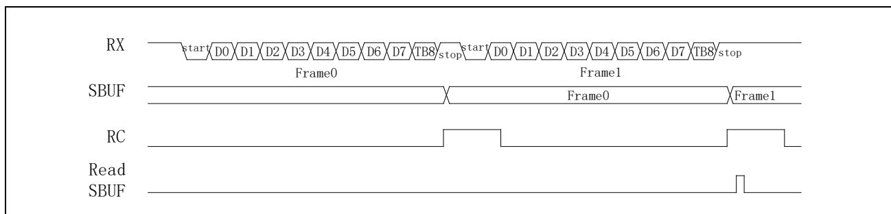
图 22-13 接收缓存
