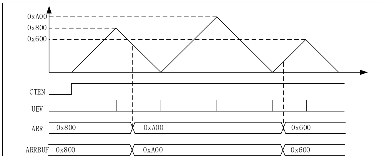
图 14-25 三角波模式下缓存无效
