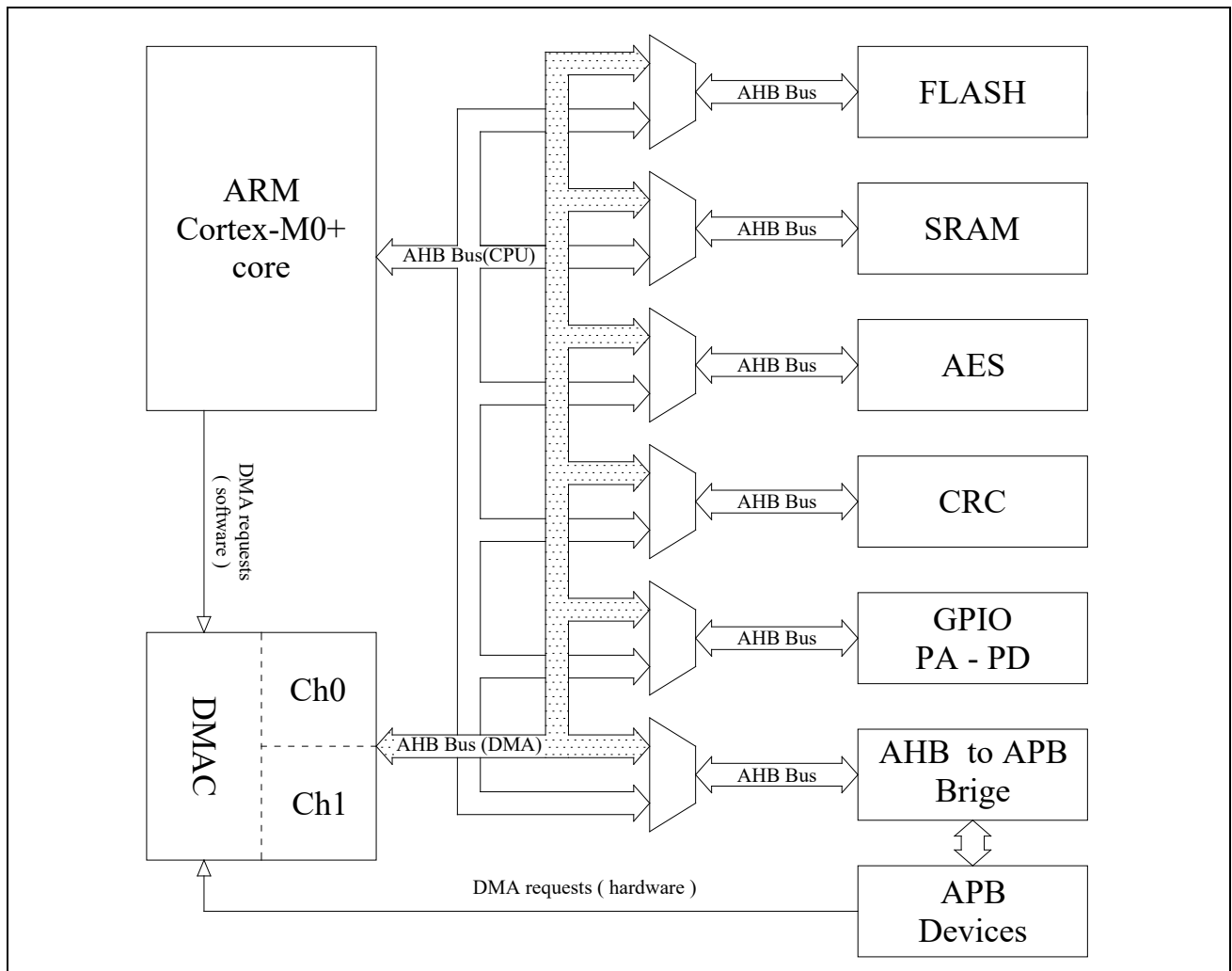
图 13-1 功能框图
