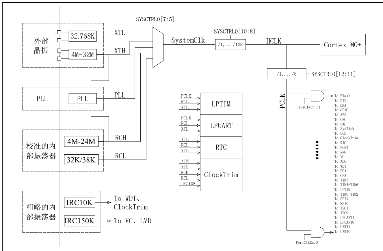
图 3-1 时钟控制模块框图
