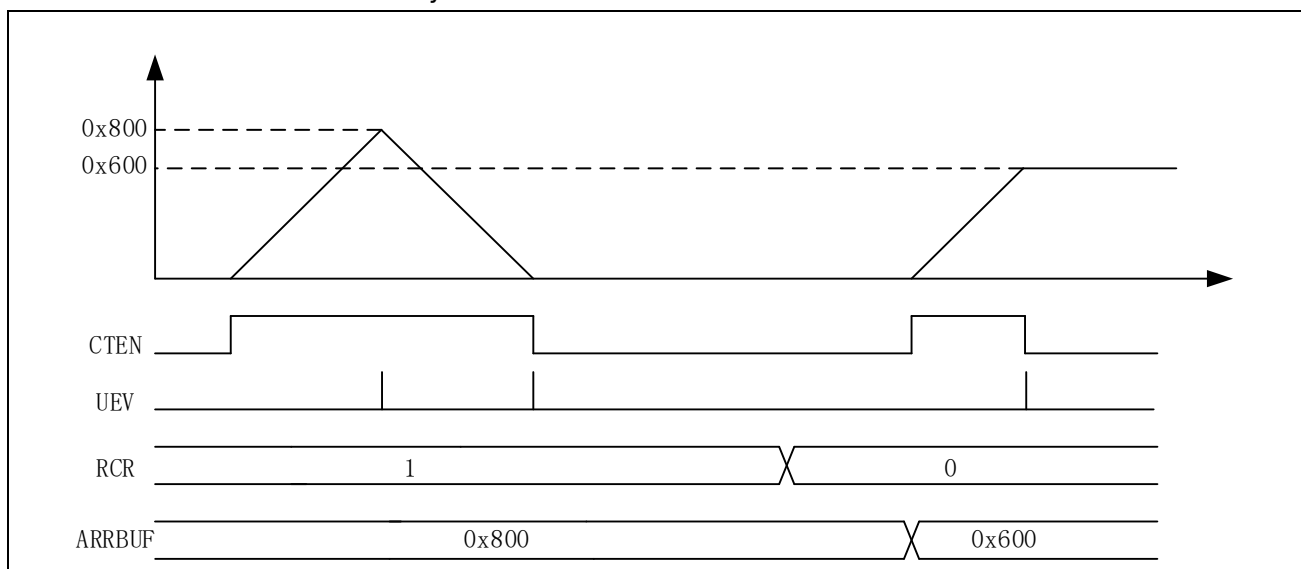
图 14-43 三角波模式单脉冲计数
