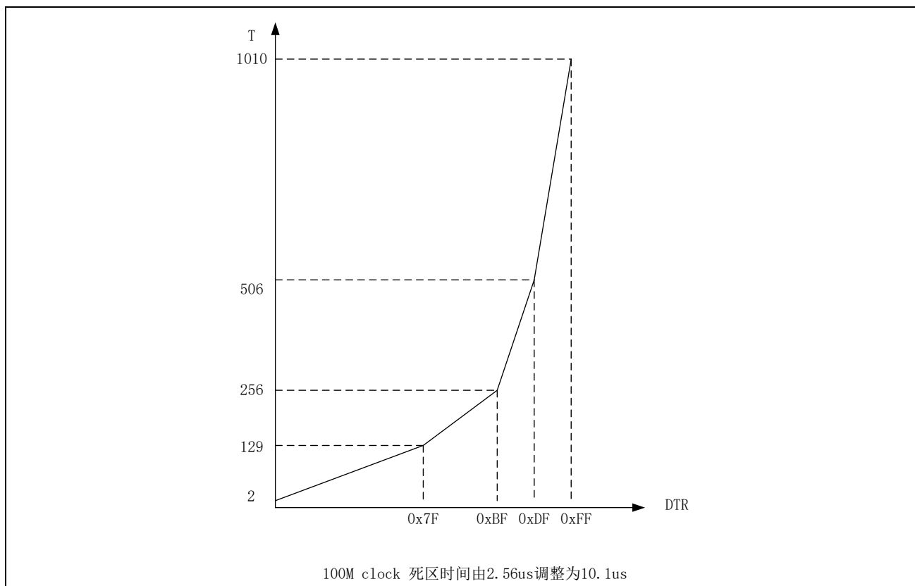
图 14-42 死区时间
