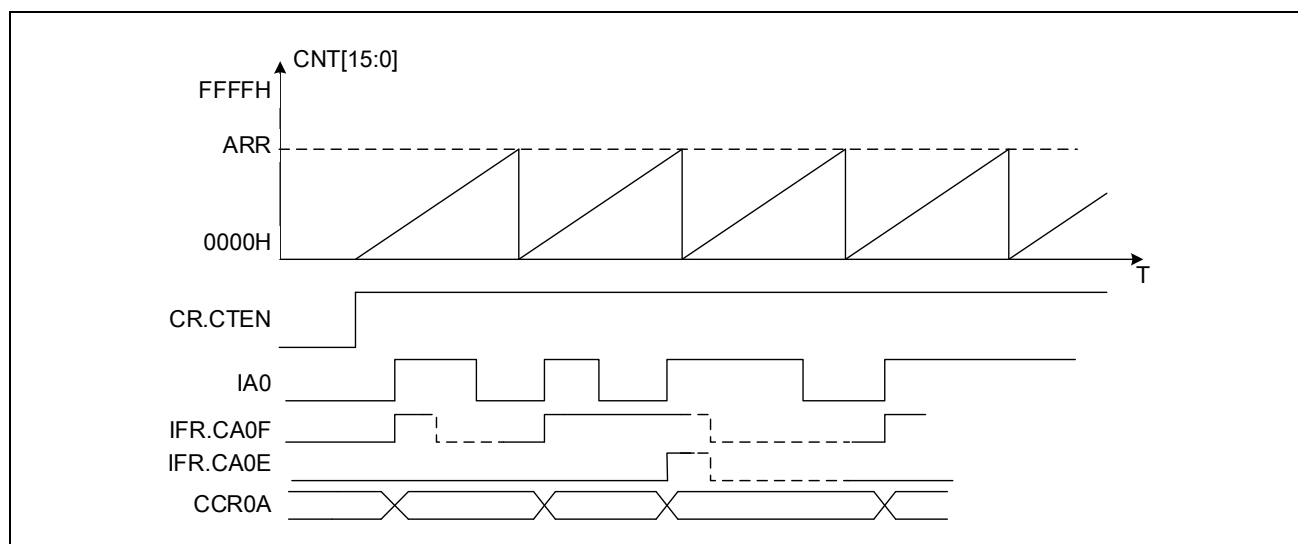
图 14-48 捕获时序图
