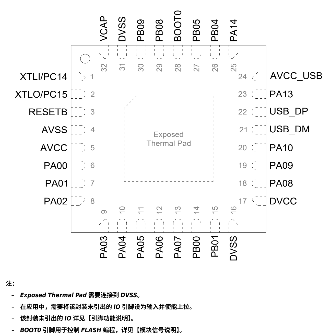
图 3-1 引脚配置图
